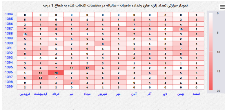
شکل ۹-۲- نمودار هیتمپ زلزله های ۱۴ ساله اخیر بشعاع ۱ درجه اطراف رومرکز زلزله ۴,۷ ونک استان اصفهان
