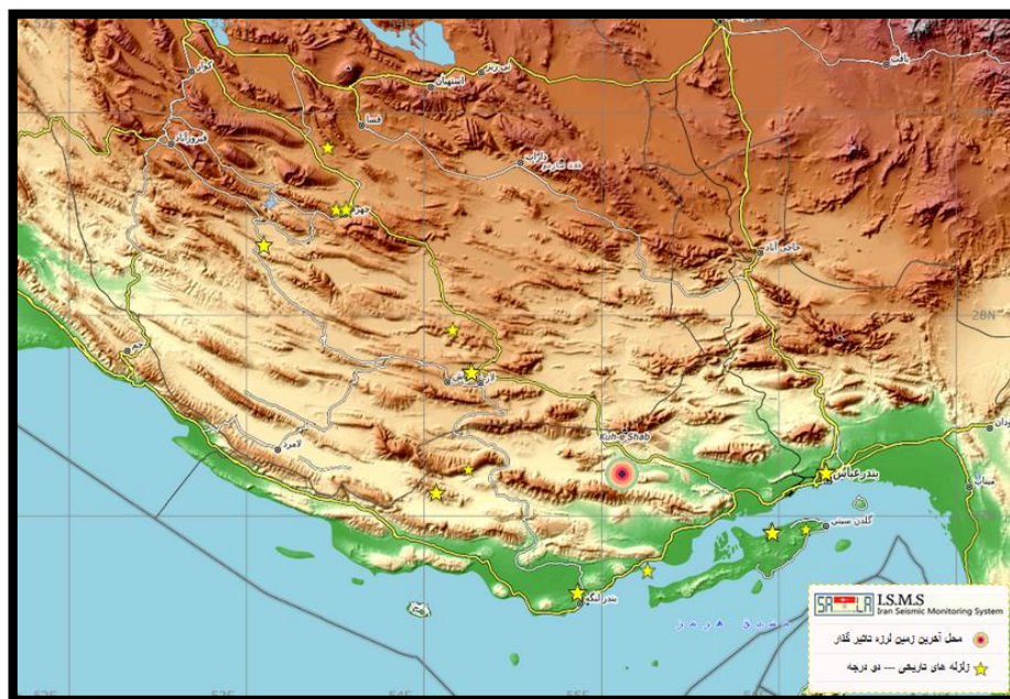
شکل ۱۱: موقعیت رومرکز زلزله ۵,۴ رویدر هرمزگان و زلزله های تاریخی اطراف آن
