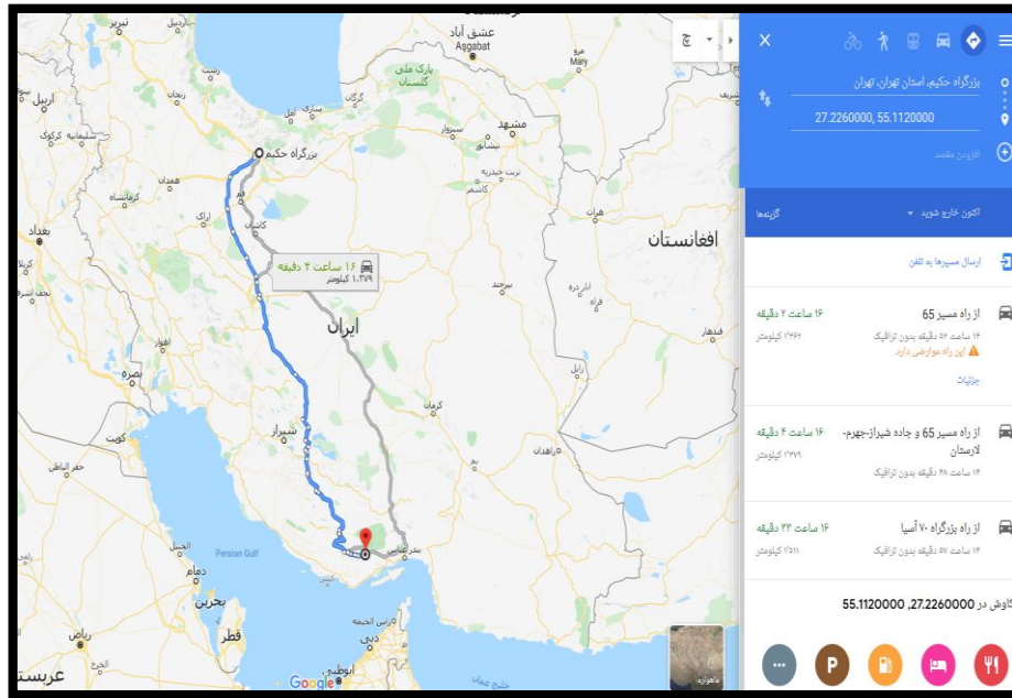
شکل ۴: موقعیت رومرکز زلزله ۵,۴ رویدر هرمزگان و مسیر دسترسی به آن از تهران
