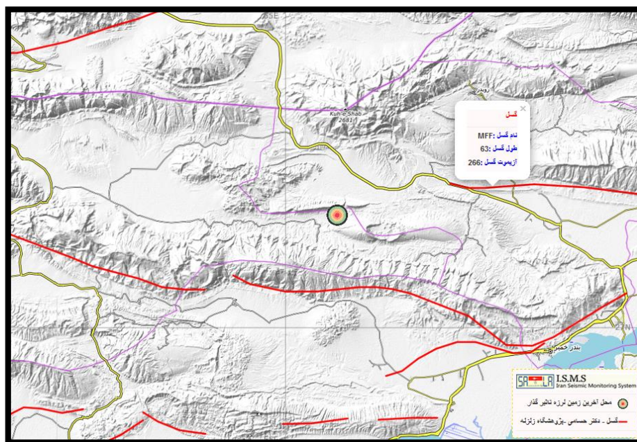
شکل ۹: موقعیت رومرکز زلزله ۵,۴ رویدر هرمزگان و گسل های اطراف آن
