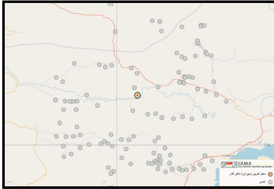
شکل ۳: موقعیت رومرکز زلزله ۵,۴ رویدر هرمزگان و آبادی اطراف آن
