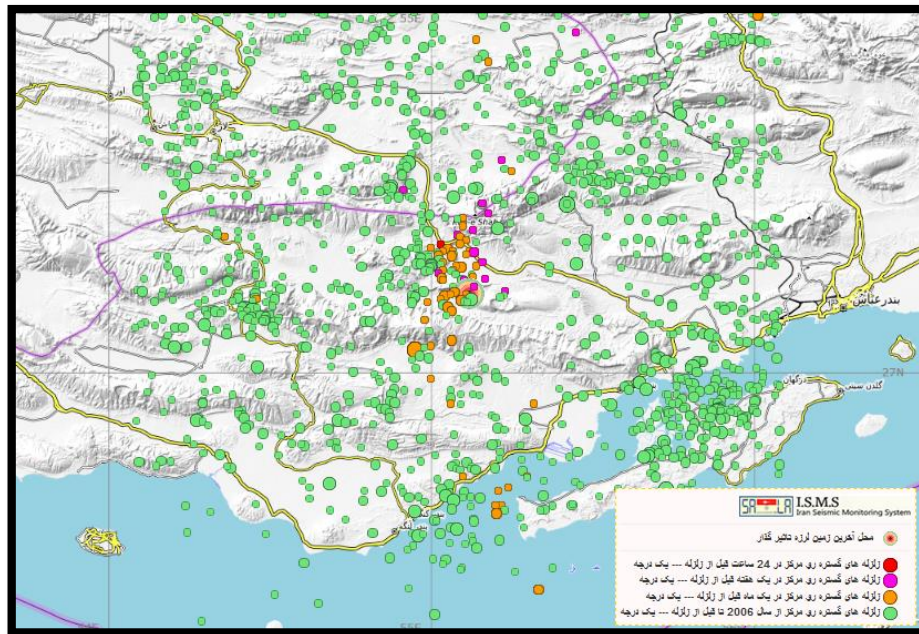
شکل ۱۳: موقعیت رومرکز زلزله ۵,۴ رویدر هرمزگان و زلزله های بالای ۲,۵ دستگاهی اطراف آن از سال ۲۰۰۶ تا زمان وقوع زلزله
