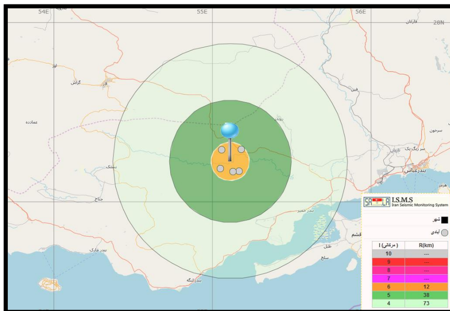
شکل ۱۶: موقعیت رومرکز زلزله ۵,۴ رویدر هرمزگان و شدت تخمینی آن (شدت موثری محاسبه نشده است)
