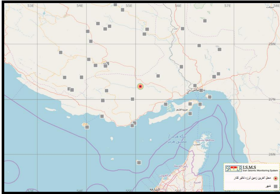
شکل ۲: موقعیت رومرکز زلزله ۵,۴ رویدر هرمزگان و شهرهای اطراف آن جدول ۴ ، فاصله مستقیم تعدادی از آبادی ها را از رومرکز زلزله نشان می دهد. جدول ۵: فاصله مستقیم مراکز جمعیتی روستائی و آبادی ها از رومرکز زلزله
