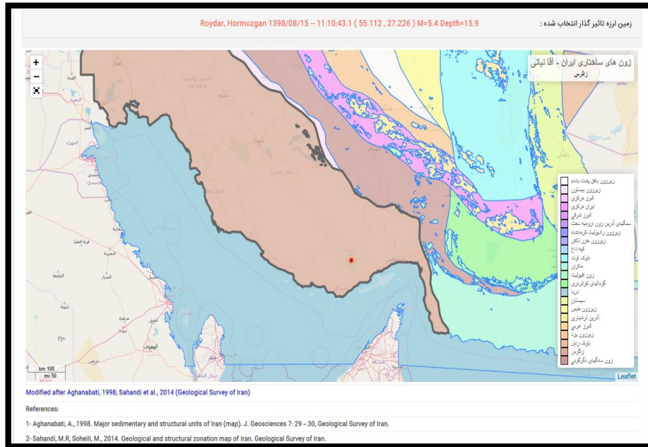
شکل ۱۰: موقعیت رومرکز زلزله ۵,۴ رویدر هرمزگان و ایالت لرزه زمین ساختی زاگرس در اطراف آن
