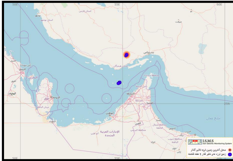
شکل ۱: موقعیت رومرکز زلزله ۵,۴ رویدر هرمزگان
