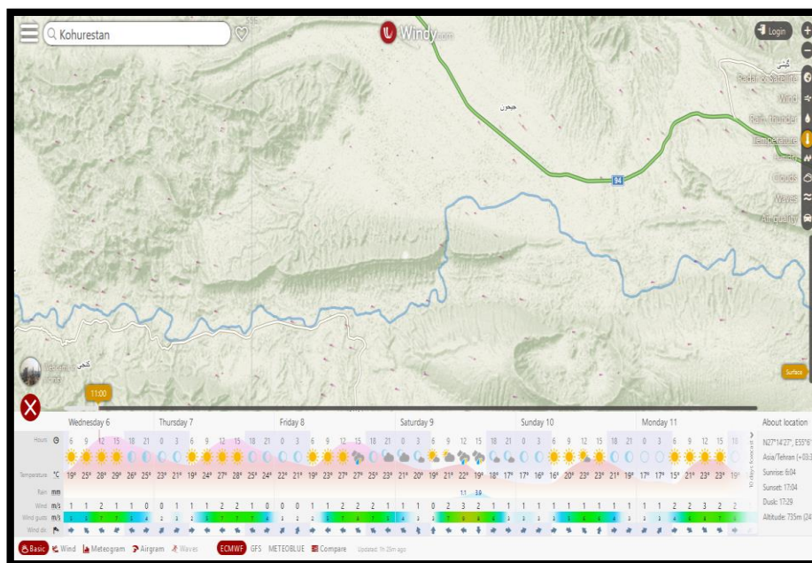
شکل ۵: موقعیت رومرکز زلزله ۵,۴ رویدر هرمزگان (نقطه وسط نقشه) اطلاعات پیش بینی هوا
