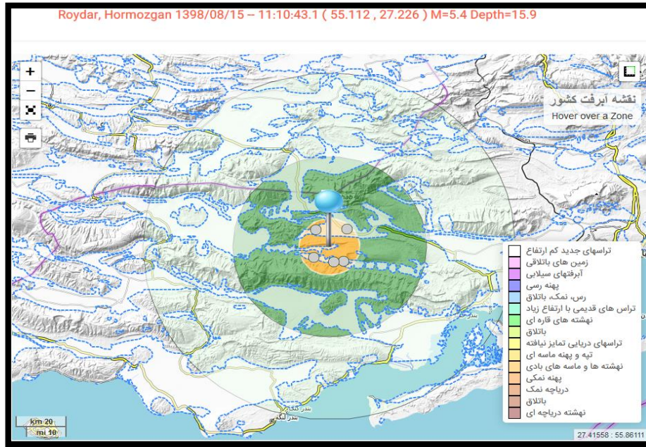
شکل ۱۷: موقعیت رومرکز زلزله ۵٫۴ رویدر هرمزگان و پهنه های گسترش آبرفت های اطراف آن
