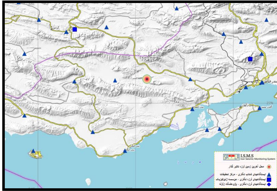
شکل ۱۵: موقعیت رومرکز زلزله ۵٫۴ رویدر هرمزگان و پراکنش ایستگاه ای شتابنگاری و لرزه نگاری
