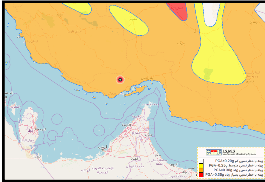
شکل ۱۸: موقعیت رومرکز زلزله ۵,۴ رویدر هرمزگان و بهینه خطر زیاد زلزله در بر گیرنده آن
