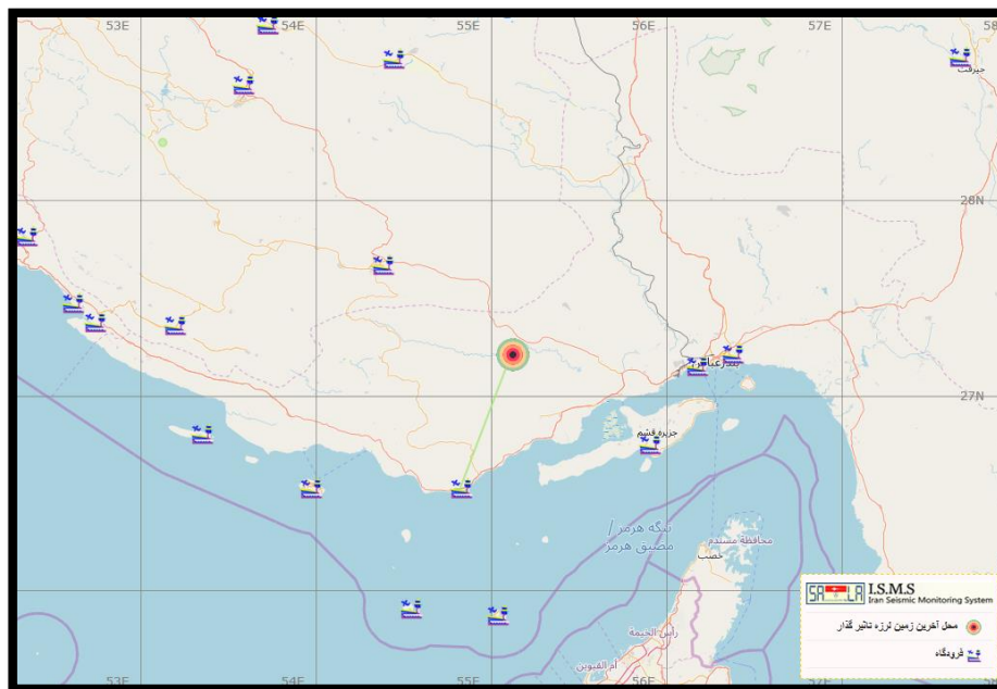
شکل ۲۱: موقعیت رومرکز زلزله ۵٫۴ رویدر هرمزگان و فرودگاه های مجاور آن
