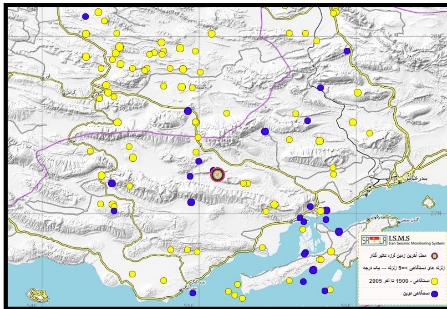
شکل ۱۲: موقعیت رومرکز زلزله ۵,۴ رویدر هرمزگان و زلزله های بالای ۵ دستگاهی اطراف آن
